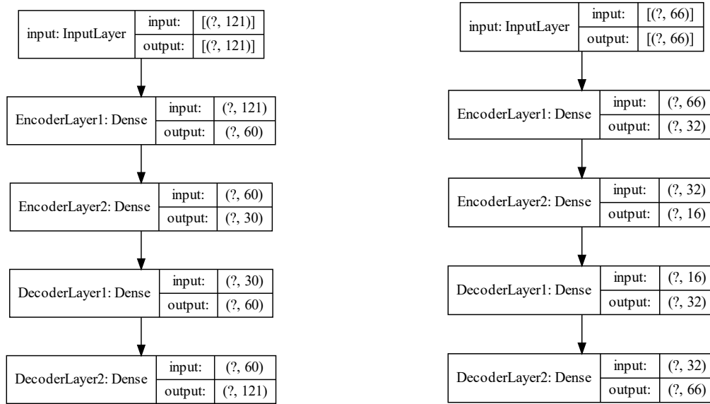
(a) NSL-KDD
