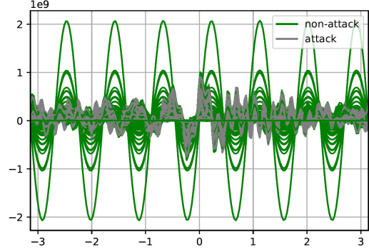
(b) CIC-IDS2017(DoS) dataset
